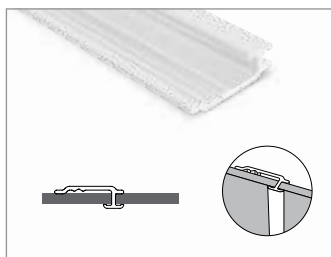
PROFILÉ DE LIAISON
